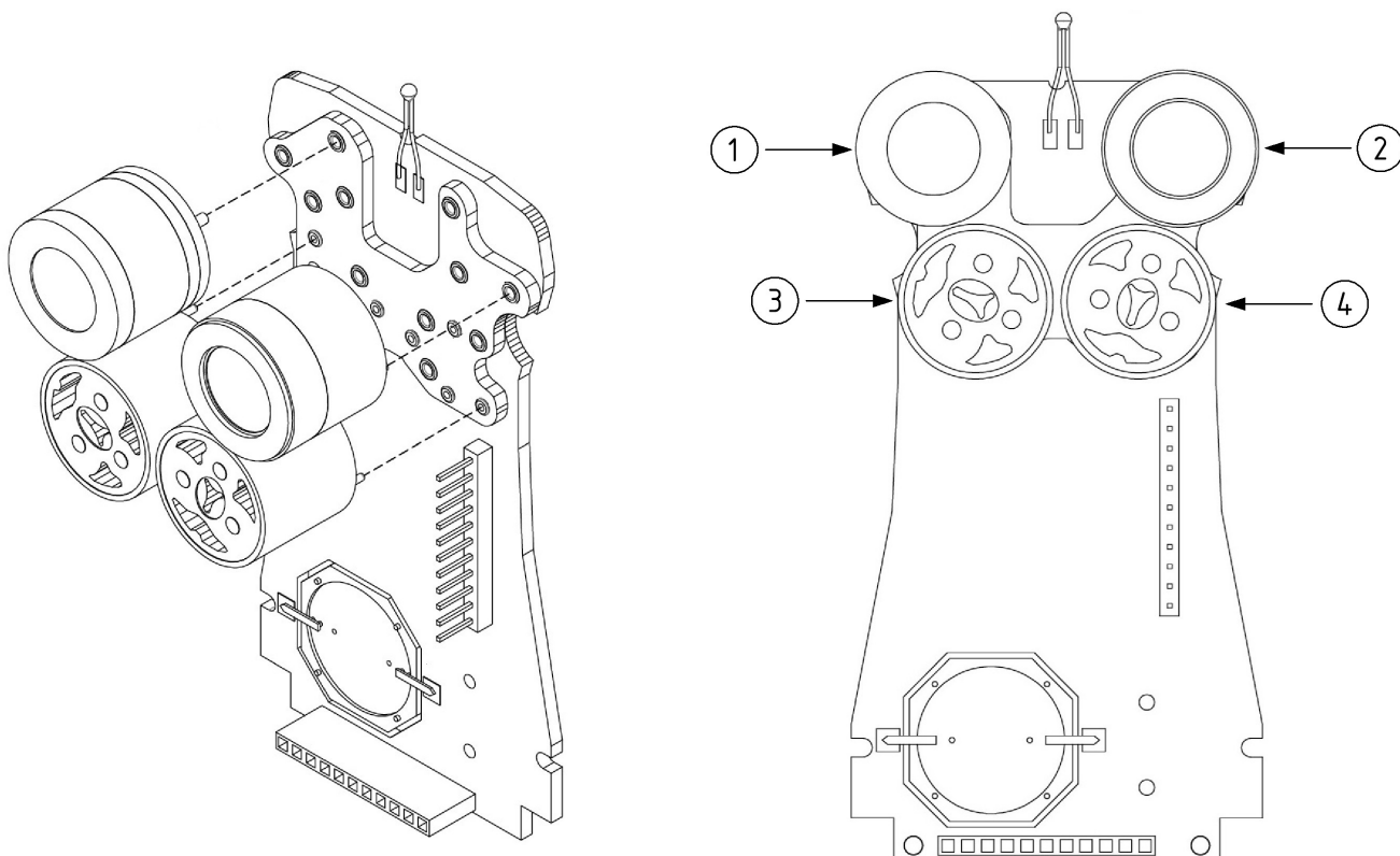
Рисунок 6 – Расположение датчиков
