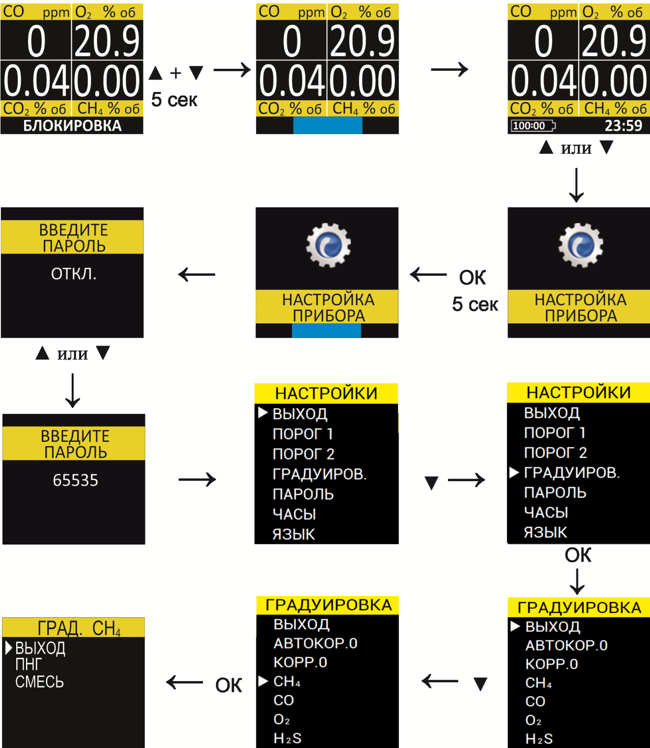
Рисунок 23 – Вход в меню градуировки метана
