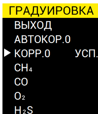
Рисунок 27 – Корректировка нуля
